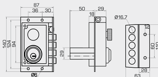
Esquema apertura derecha
